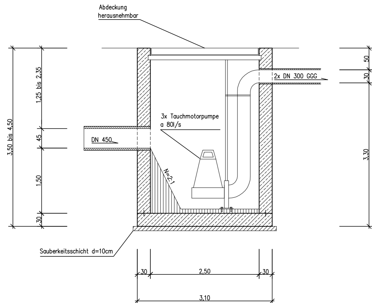
Schnitt A-A M=1:50
