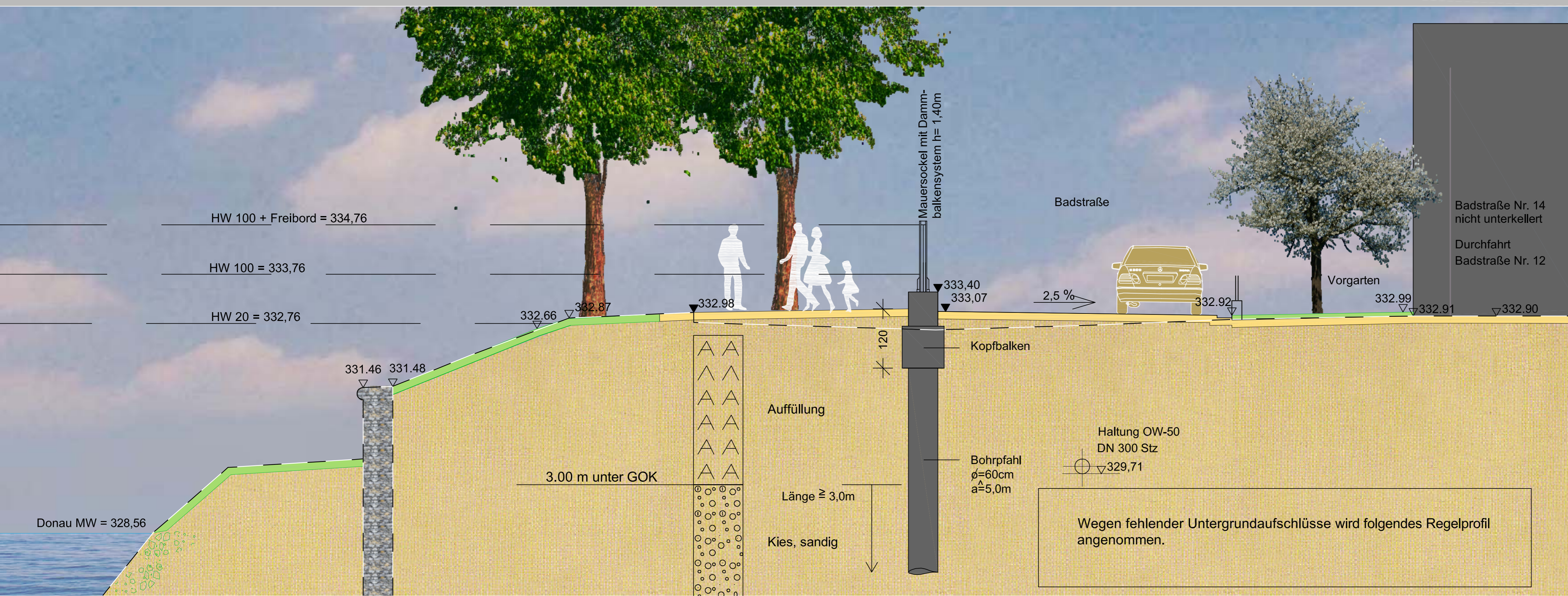
SCHNITT M 1:50
