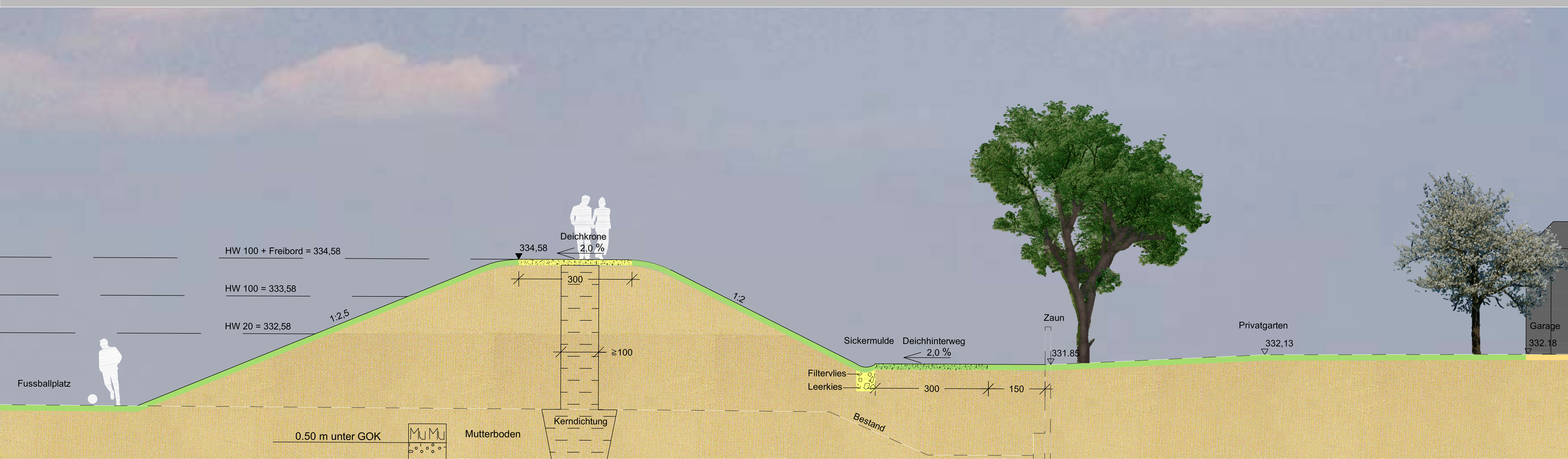
SCHNITT M 1:50
