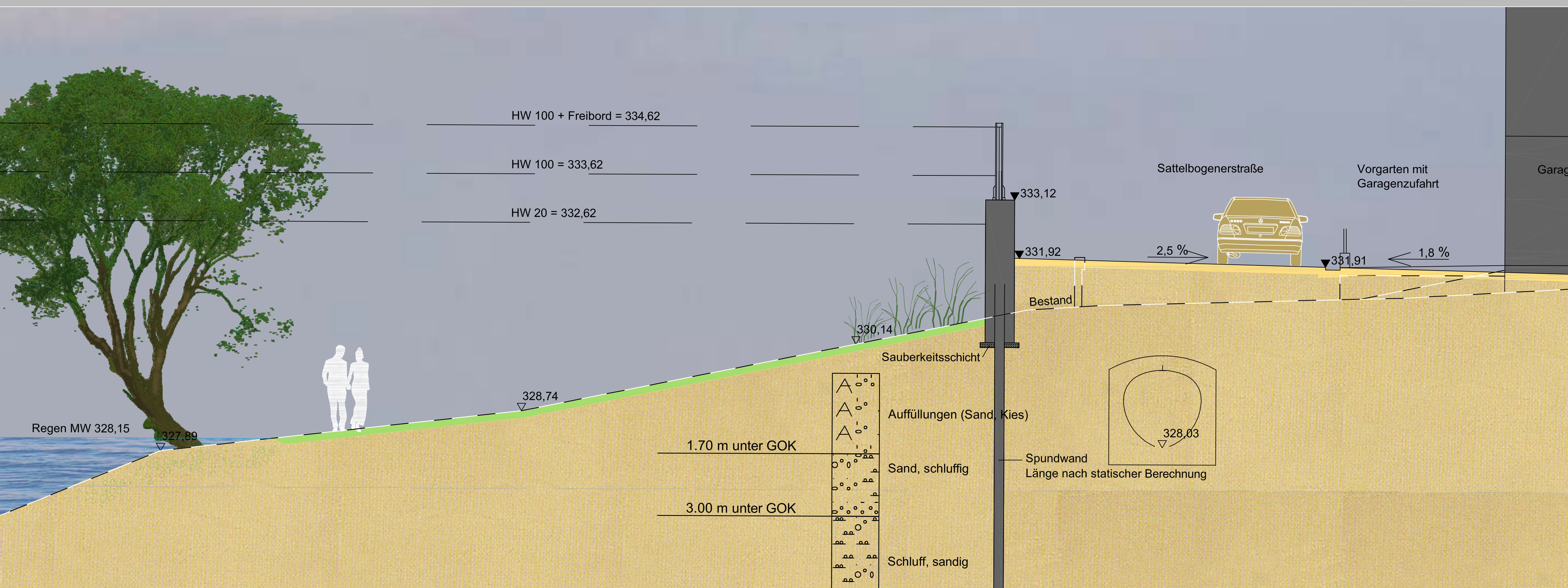
SCHNITT M 1:50
